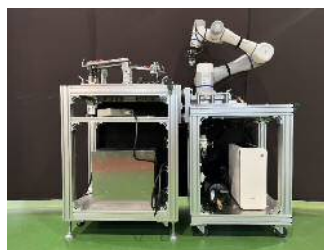
三機オリジナル商品 協働ロボット台車連結 ガッチャンコ
